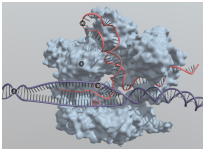
CRISPR/Cas9
