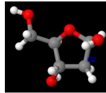
Deoxyribose
