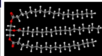
Triglyceride
