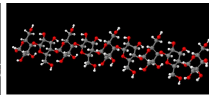
Cellulose
